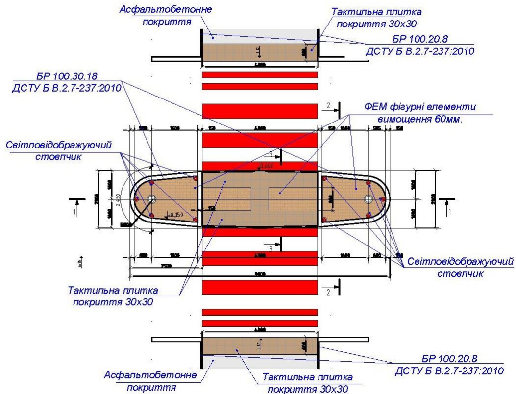
План острівця безпеки М1:100
