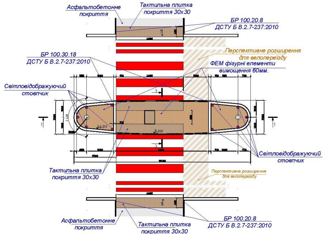
План острівка безпеки з смугою для велосипедистів М1:100
